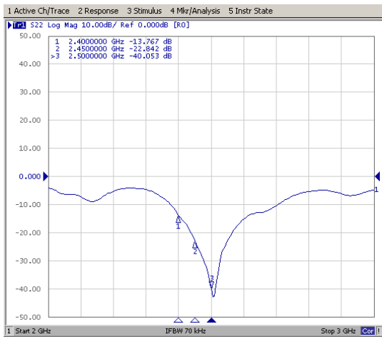
Обратные потери
