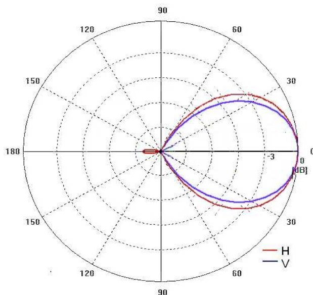
Рис.3 Диаграмма направленности антенного комплекса АКМ-900(Н)
