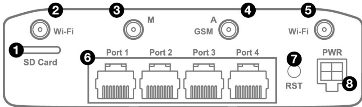
Рис. 2. Вид сзади
