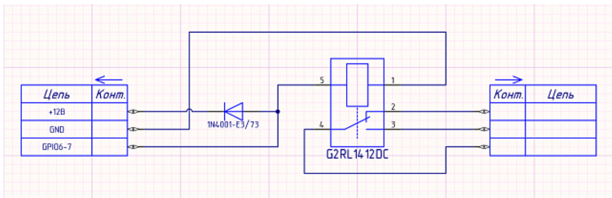
Рис. 15. Схема для подключения электромагнитных реле к GPIO6, GPIO7
