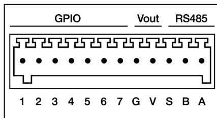
Рис. 7. Интерфейсный разъём
