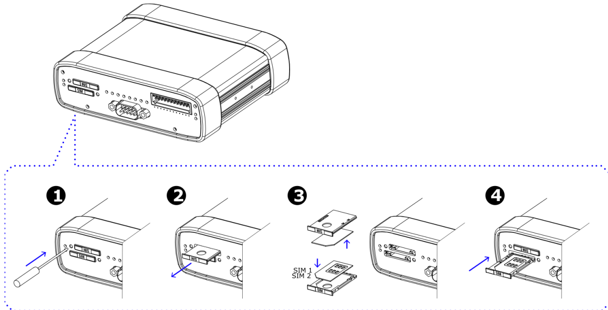
Рис. 9. Установка SIM-карт
