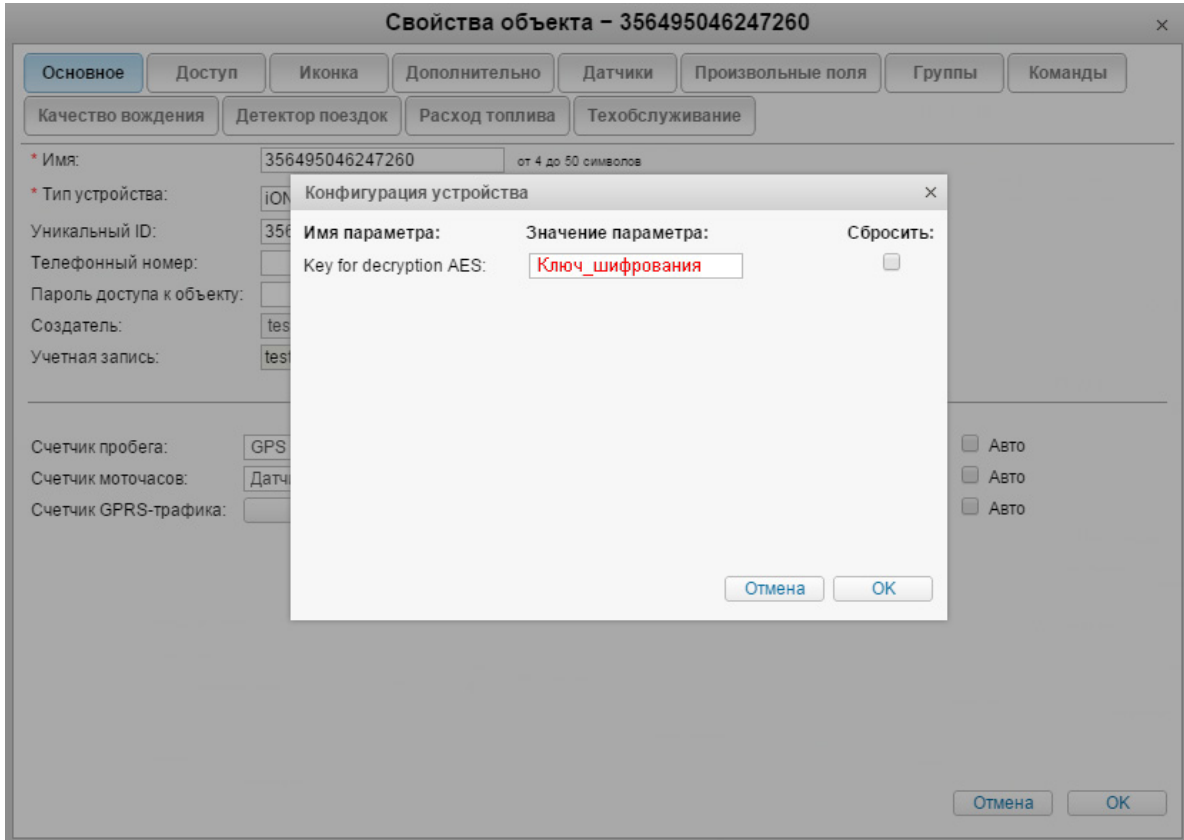
Рис. 4. Сервис Wialon, ввод ключа шифрования
