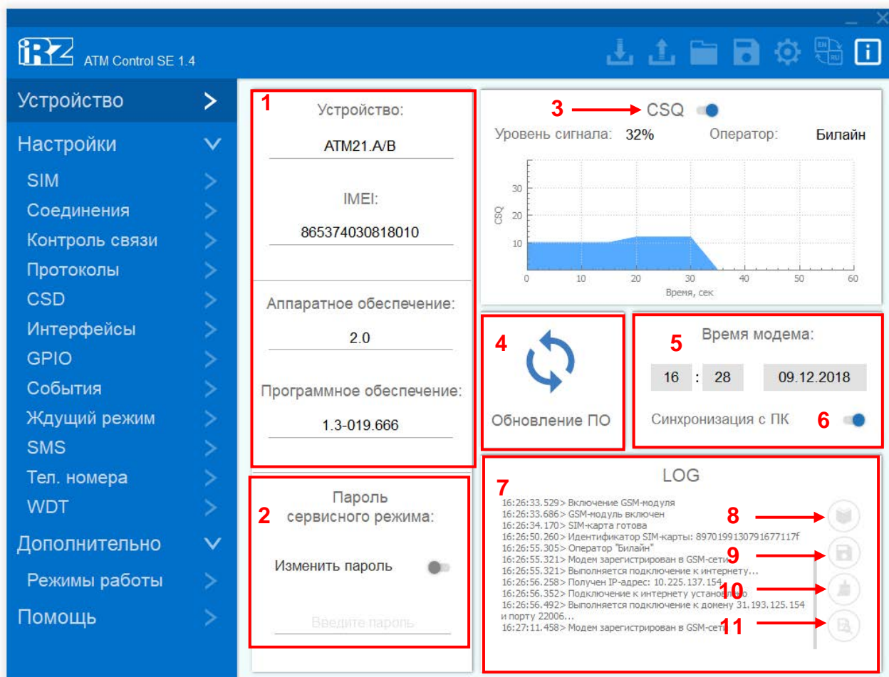
Рис. 2.2 Вкладка «Устройство»
